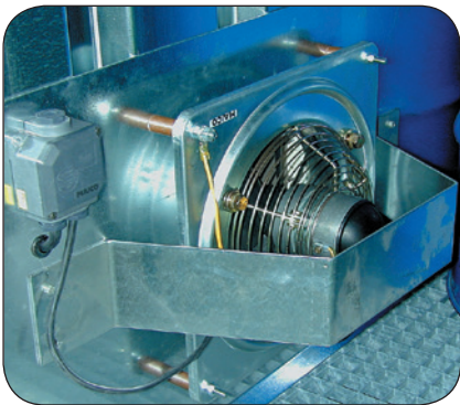
Zubehör: Technische Zwangsentlüftung, ex-geschützt, Artikel-Nr. H61-9006-C, für die aktive Lagerung von entzündbaren Stoffen
